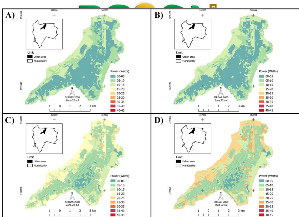
Figura 6 – Potencial eólico estimado com velocidade média a 10, 20, 30 e 40 metros de altura.
