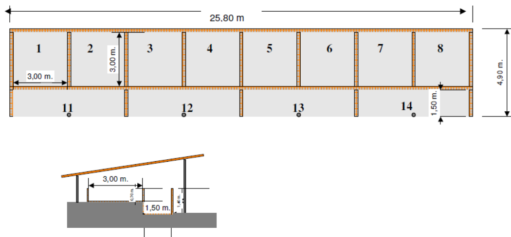
FIGURA 3 - PLANTA BAIXA E CORTE DAS CONSTRUÇÕES DAS CÂMARAS DE INCORPORAÇÃO E COMPOSTAGEM.
